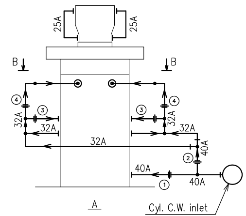
6UEC50LSJ Piping diagram of cylinder cooling water (Uniflow cooling) シリンダ冷却水管線図 (ユニフロー冷却) 11-1/17
