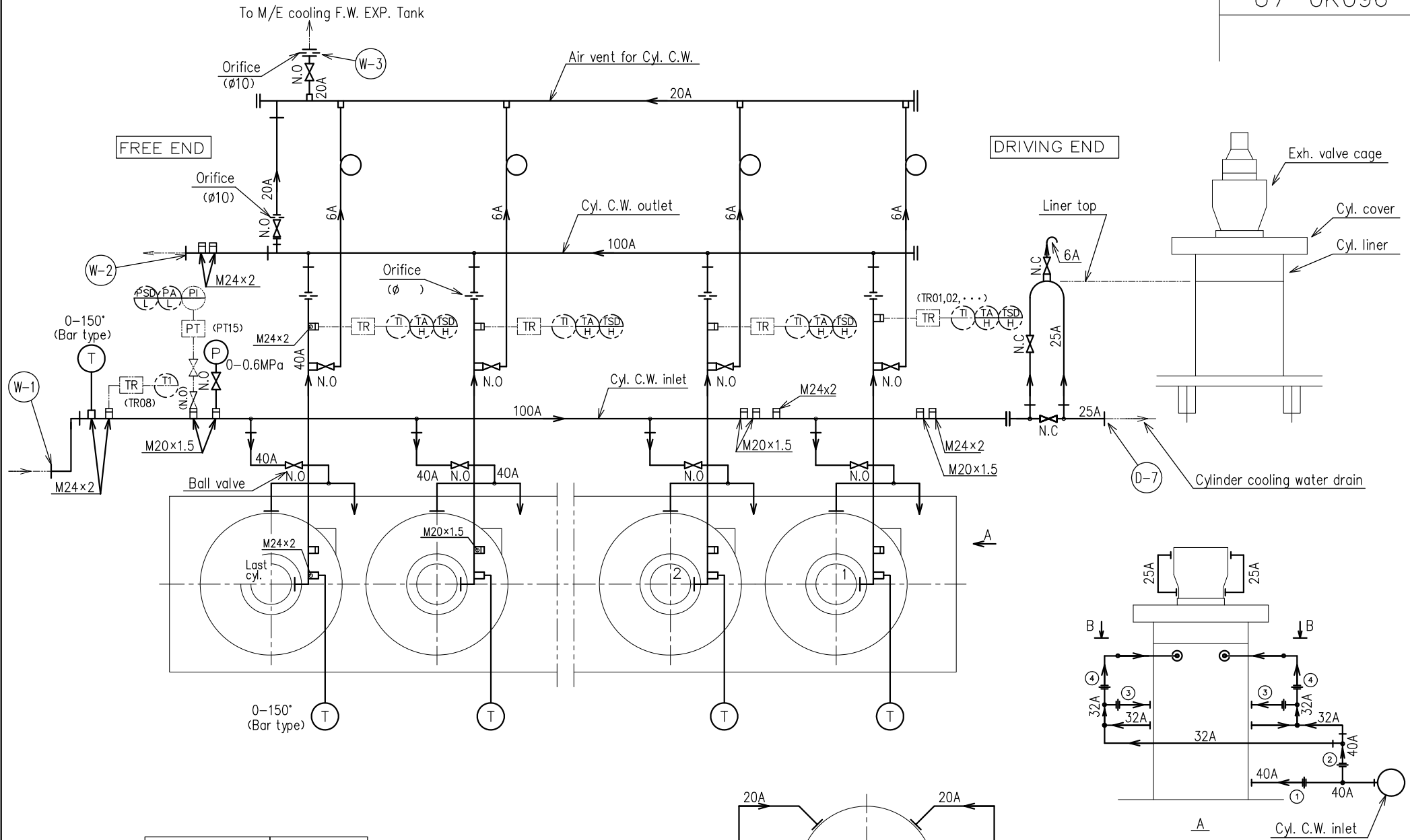
6UEC50LSJ Piping diagram of cylinder cooling water (Uniflow cooling) シリンダ冷却水管線図 (ユニフロー冷却) 11-1/17
