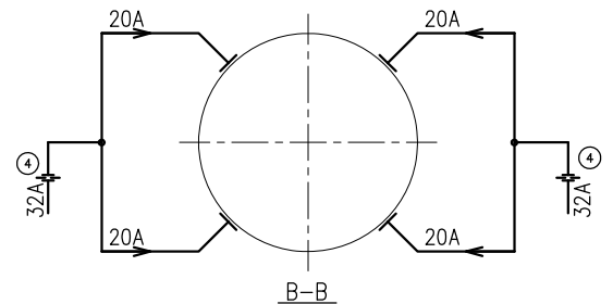
6UEC50LSJ Piping diagram of cylinder cooling water (Uniflow cooling) シリンダ冷却水管線図 (ユニフロー冷却) 11-1/17
